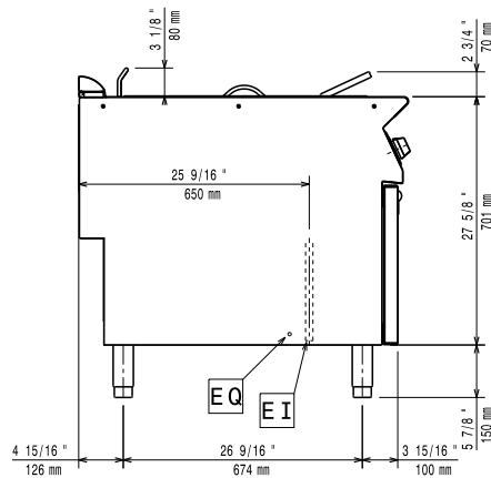
Oldalnézet
